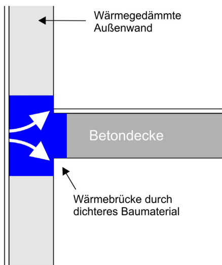
Abb. 7: An tragenden Bauteilen mit geringer Materialdichte und damit guter Wärmeleitung (z.B. Beton) ergeben sich Wärmebrücken, die Kondenswasserbildung begünstigen.
